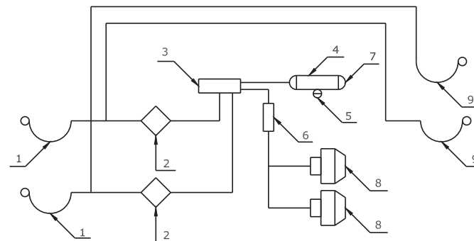
Рис. 3 Схема пневматической двухпроводной тормозной системы.
