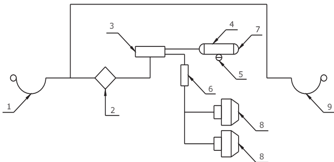
Рис. 2 Схема однопроводной пневматической тормозной системы.
