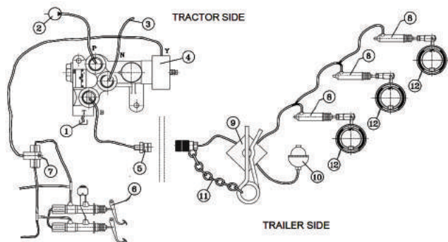
Рис. 5. Схема тормозной гидравлической системы: СО СТОРОНЫ ТРАКТОРА
